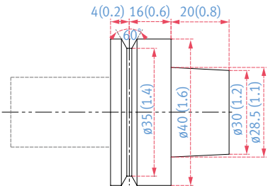
DIN 69893 HSK-E40
